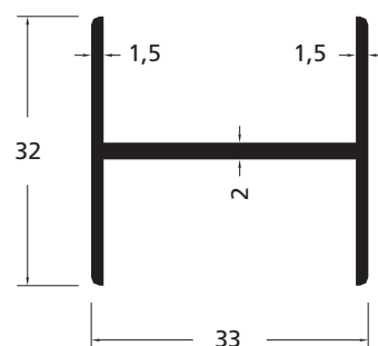
Artikelnummer 171651 (schaal 1:1)
