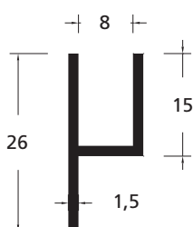
Artikelnummer 170097 (schaal 1:1)
