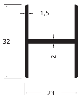
Artikelnummer 171650 (schaal 1:1)
