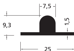
Artikelnummer 179320 (schaal 1:1)
