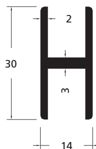
Artikelnummer 171249 (schaal 1:1)
