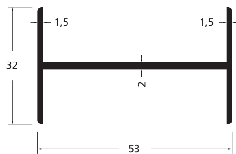
Artikelnummer 171651 (schaal 1:1)
