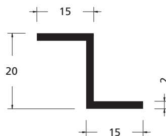
Artikelnummer 173609 (schaal 1:1)
