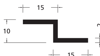
Artikelnummer 173610 (schaal 1:1)
