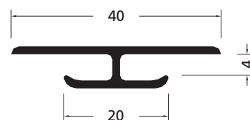
Artikelnummer 172358 (schaal 1:1)
