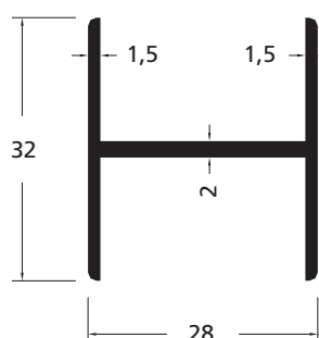
Artikelnummer 171650 (schaal 1:1)
