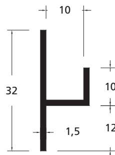
Artikelnummer 170155 (schaal 1:1)
