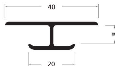
Artikelnummer 172360 (schaal 1:1)
