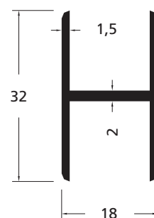
Artikelnummer 171649 (schaal 1:1)
