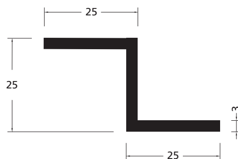
Artikelnummer 173655 (schaal 1:1)
