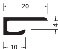
Artikelnummer 172357 (schaal 1:1)
