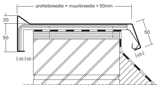
Muurafdekker Roval type A
