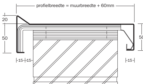
Muurafdekker Roval type B
