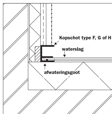
Schematische weergave van buitengevelisolatie
