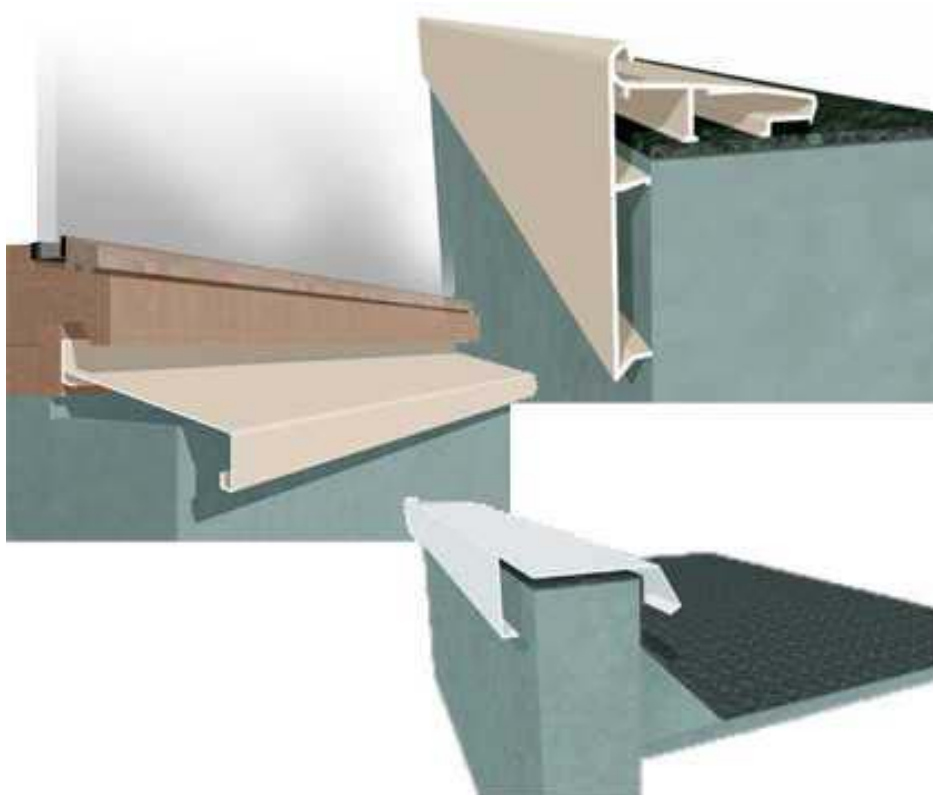
Enkele voorbeelden van waterslagen en dakranden
