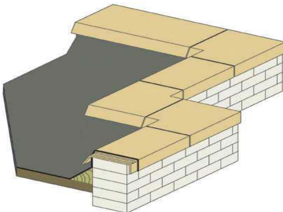
Dakrand uit gezette plaat
