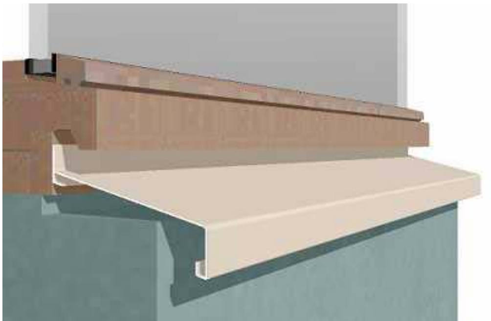
Waterslag van geëxtrudeerd profiel
